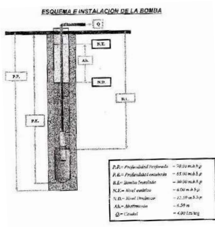
Perfil del pozo
